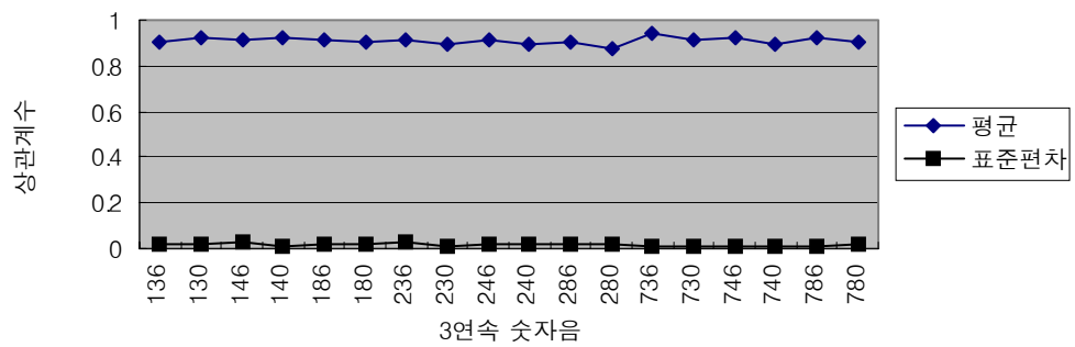
그림 7. 상관계수의 평균과 표준편차
