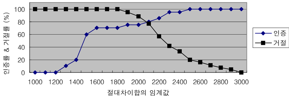
그림 10. 절대차이합 임계값의 변화에 따른 인증률과 거절률의 관계
