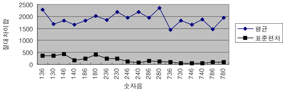
그림 6. 절대차이합의 평균과 표준편차
