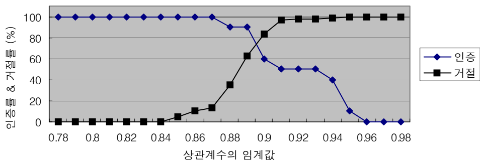
그림 11. 상관계수 임계값의 변화에 따른 인증률과 거절률의 관계
